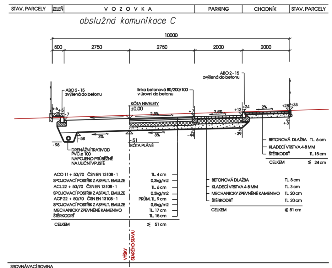
Obslužné komunikace C - šířka 10 m
