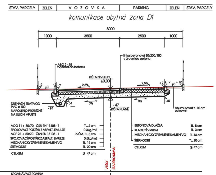
Zklidňené komunikace D - šířka 8 m
