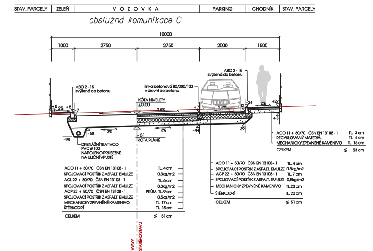
Vzorové příčné řezy Obslužné komunikace C - šířka 10 m
