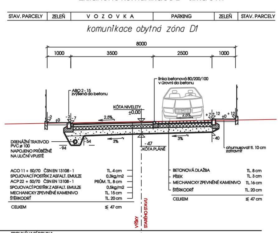
Zkldňné komunikace D - šířka 8 m
